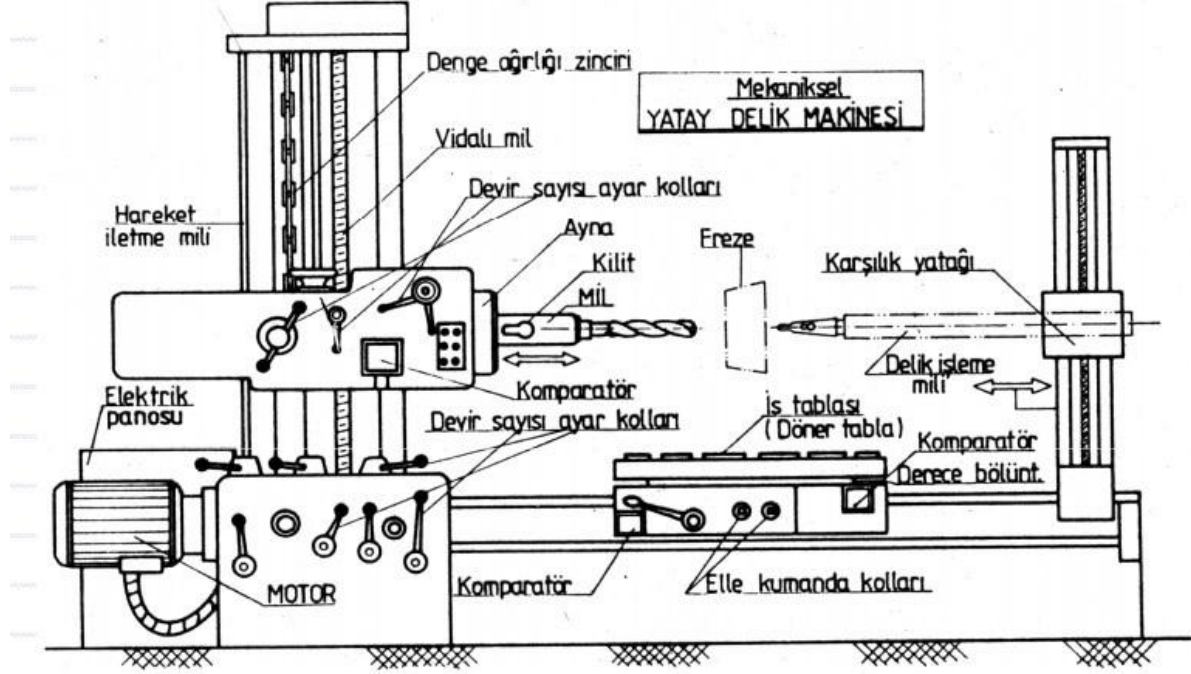
Yatay delik rezgahı ve kısımları
